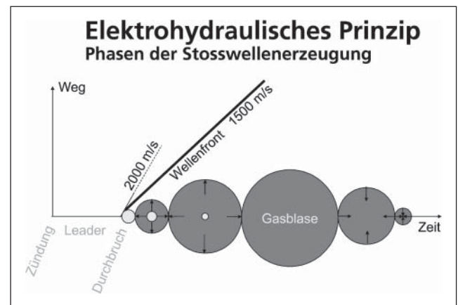
Abbildung 9: Die Phasen der elektrohydraulischen Stoßwellenerzeugung sind auf der Zeitachse dargestellt. Nach Anlegen der Hochspannung an die Elektrodenansätze entwickelt sich zunächst mit Verzögerung ein sog. „Leader“, der den Weg des Funkens bestimmt. Sobald eine leitende Verbindung zwischen den Spitzen besteht, fließt die gespeicherte elektrische Energie über den Funken und heizt die Strecke explosionsartig auf. Nur unmittelbar nach dem Durchbruch dehnt sich die Blase mit Überschallgeschwindigkeit aus (ca. 2000 m/s). Sobald die Ausbreitung der Plasmablase unter die Schallgeschwindigkeit (ca. 1500 m/s) sinkt, löst sich die Stoßwelle von der Blase ab. Unabhängig von der Stoßwelle dehnt sich die Blase weiter aus und kollabiert nach ca. 3 Millisekunden (ms), lange nachdem die Stoßwelle sich abgelöst hat.
